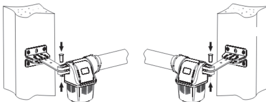
Upevnění ramene pohonu na přední konzoli.
