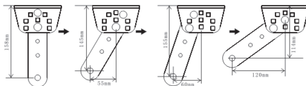
Upevnění úhlu předního oka
