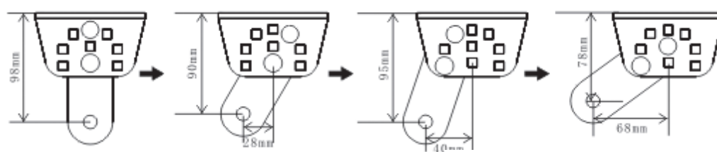
Upevnění úhlu předního oka
